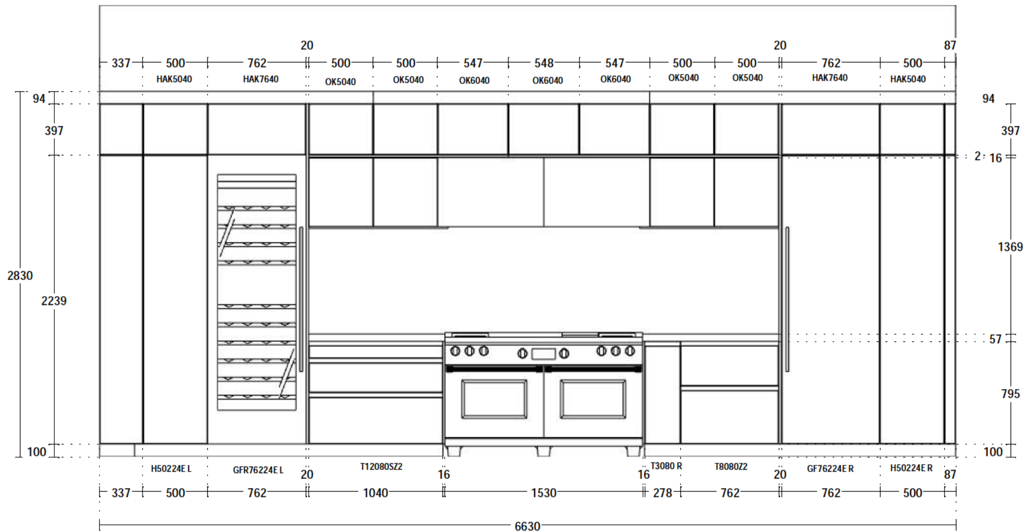
ELEVATION A
