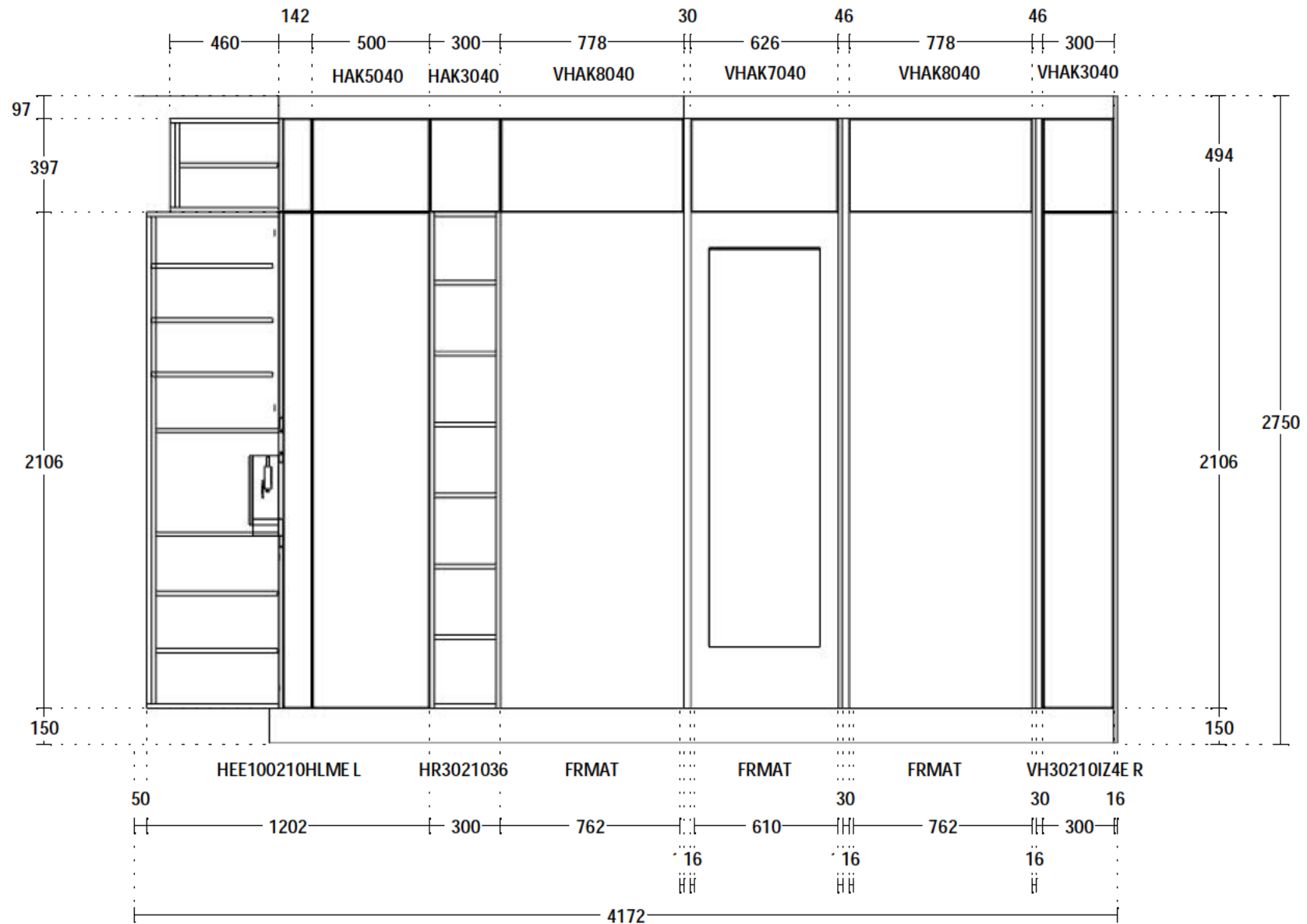
ELEVATION B
