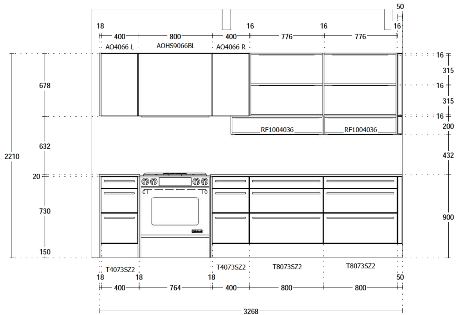
ELEVATION A
