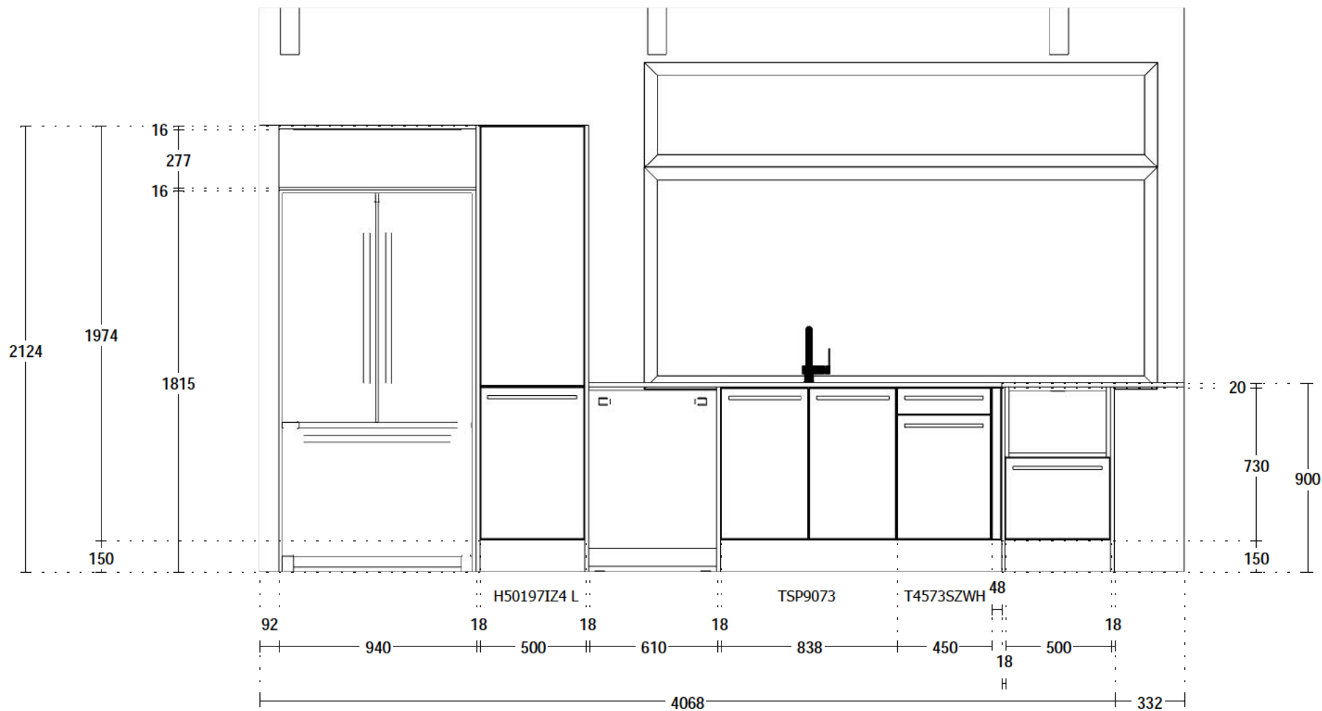
ELEVATION B
