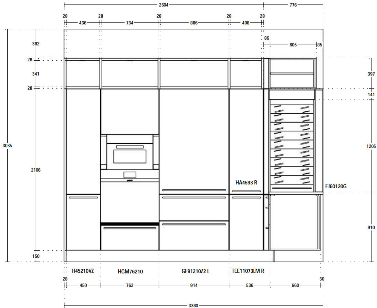
ELEVATION A
