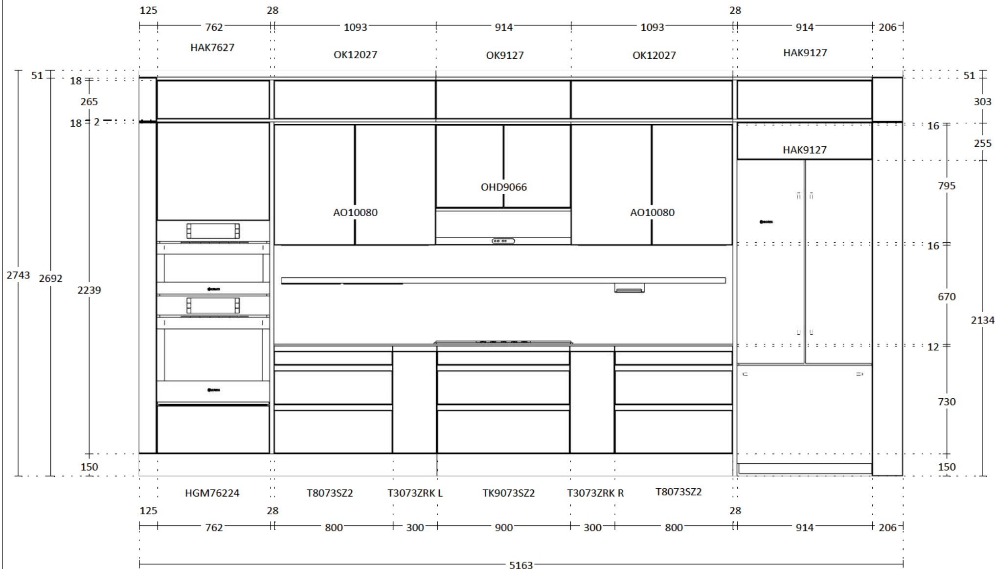
ELEVATION A
