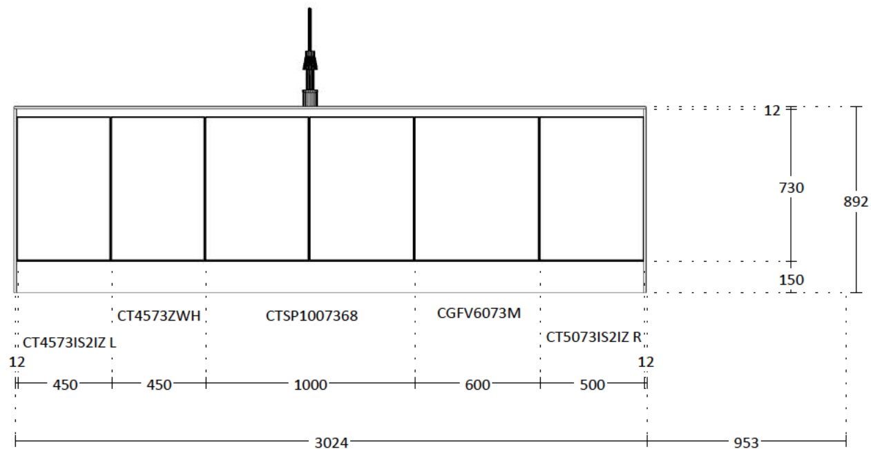
ELEVATION B
