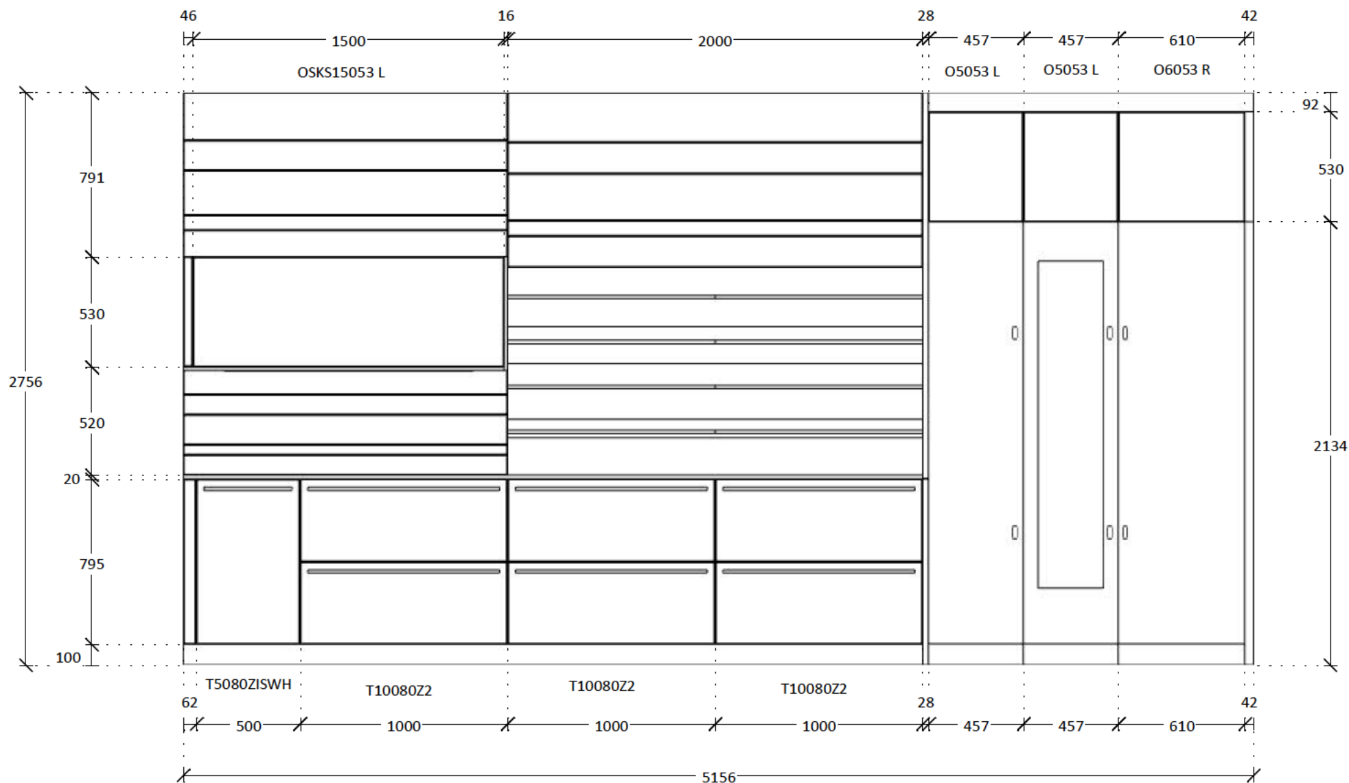
ELEVATION A
