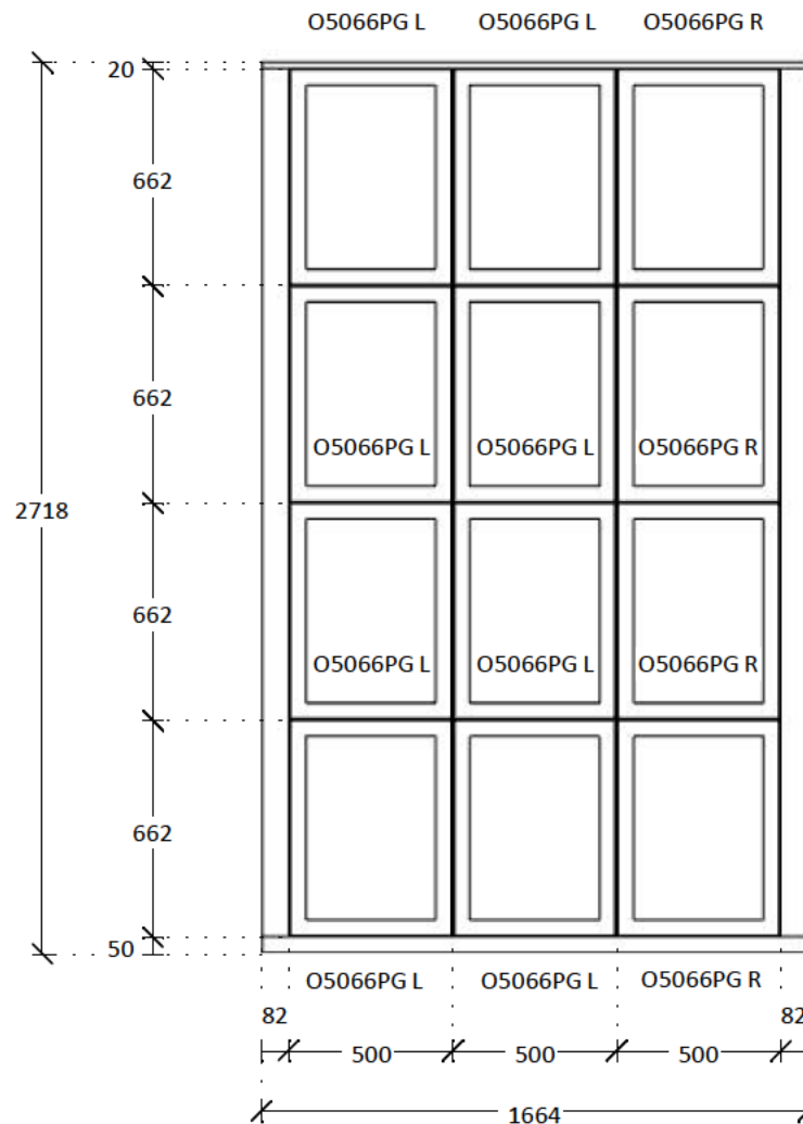
ELEVATION E
