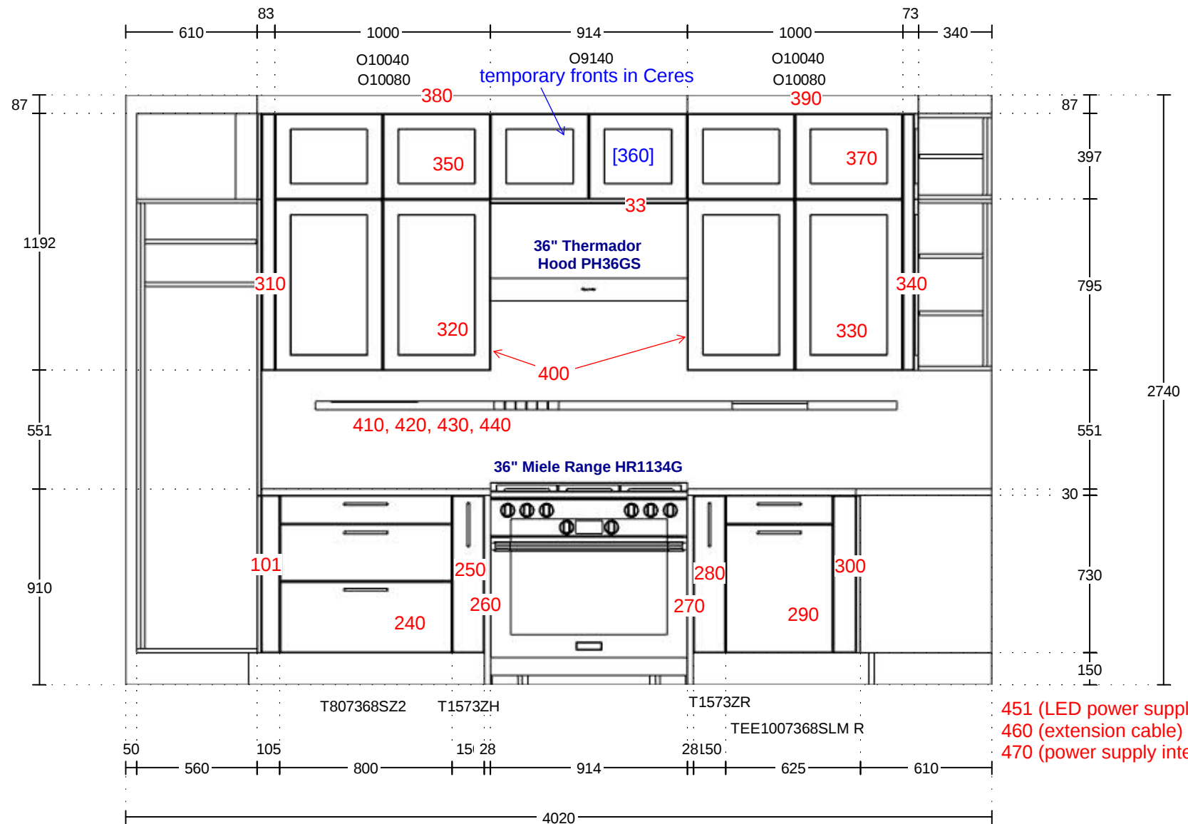
ELEVATION B
