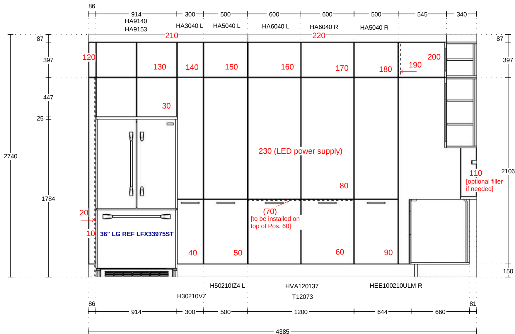
ELEVATION A
