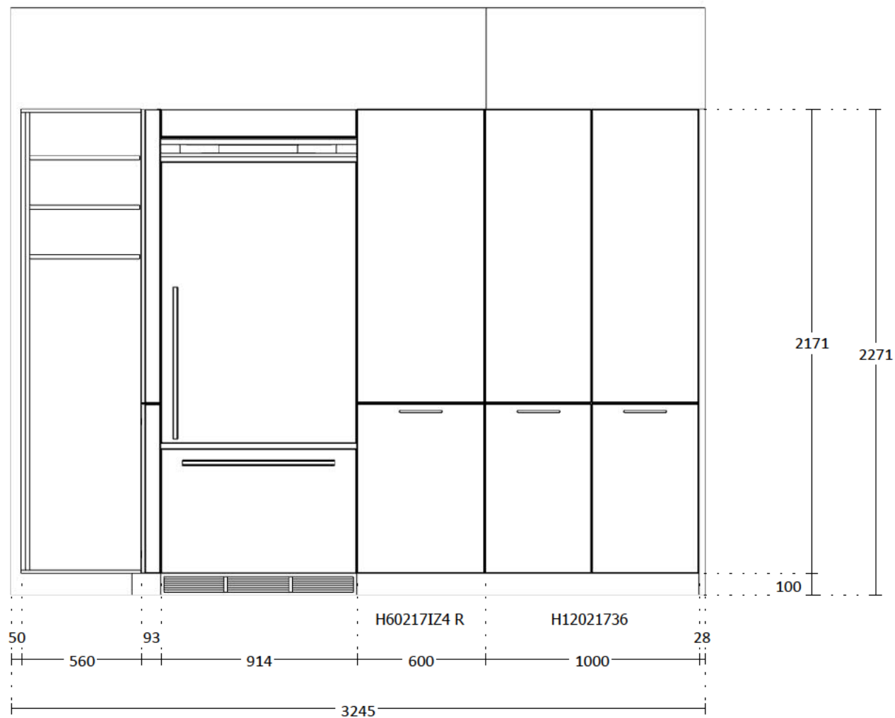
ELEVATION B
