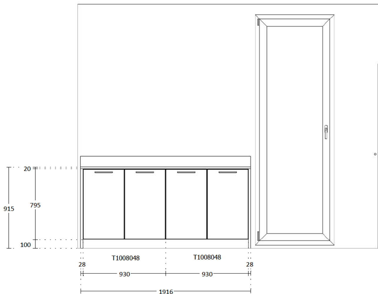
ELEVATION E
