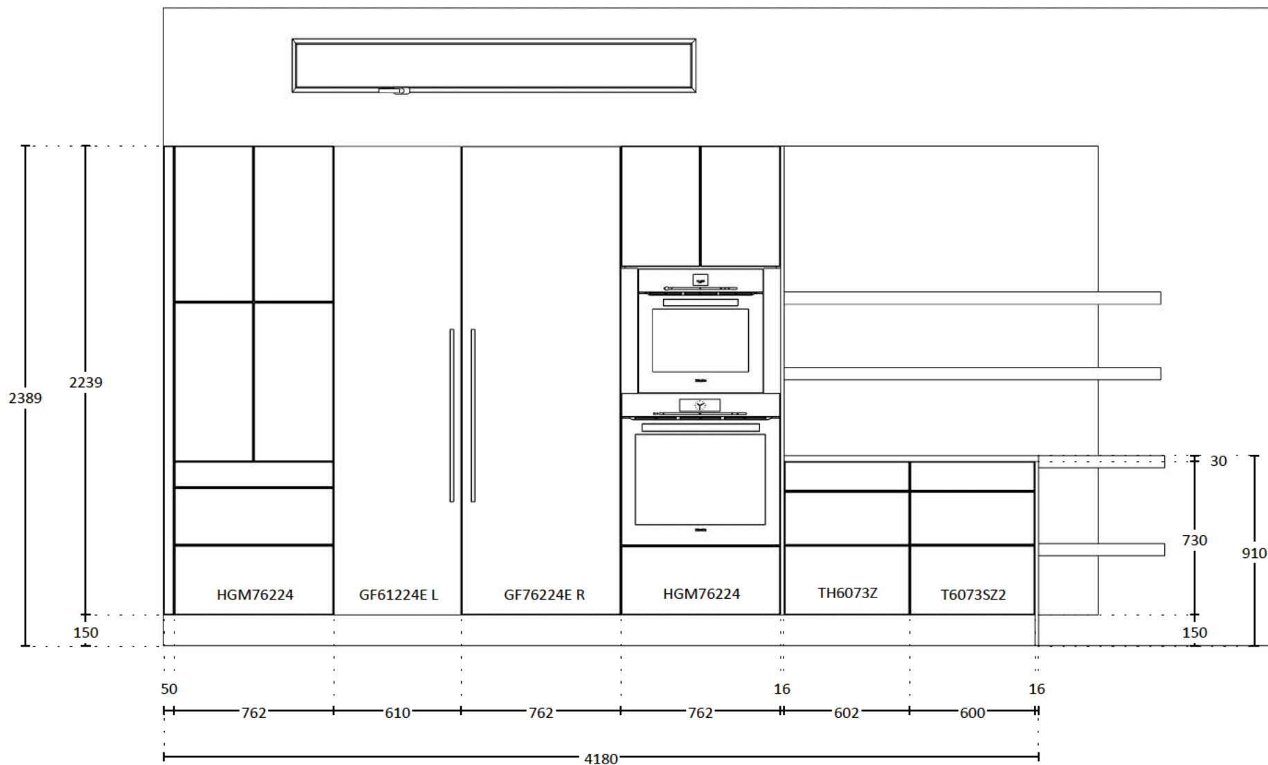
ELEVATION B
