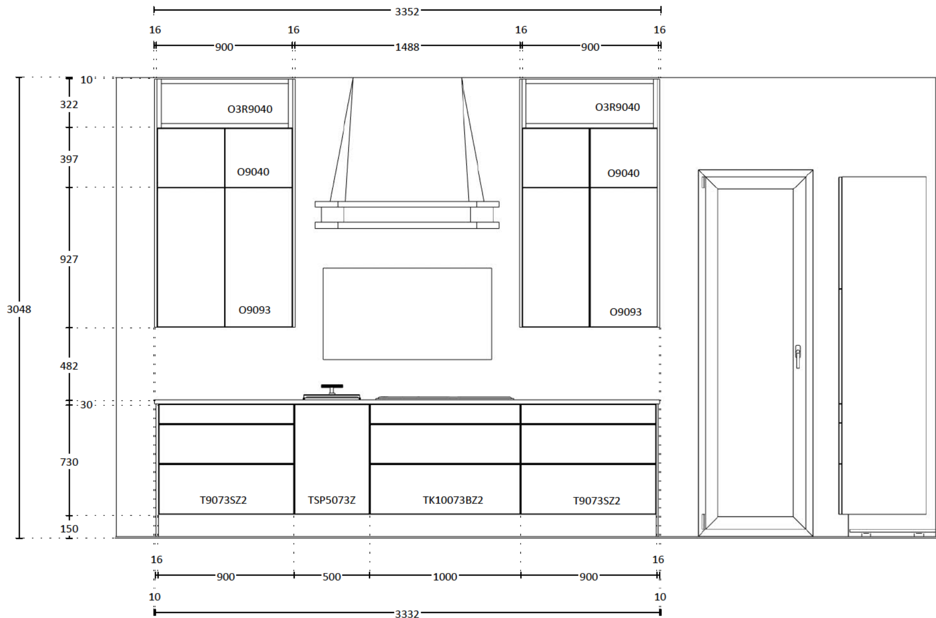
ELEVATION A
