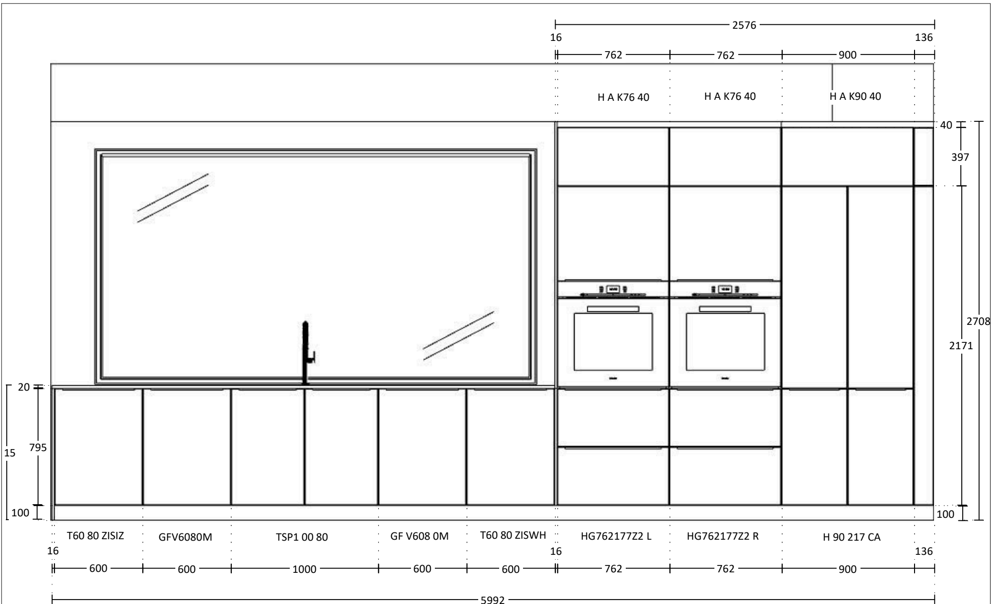
ELEVATION A
