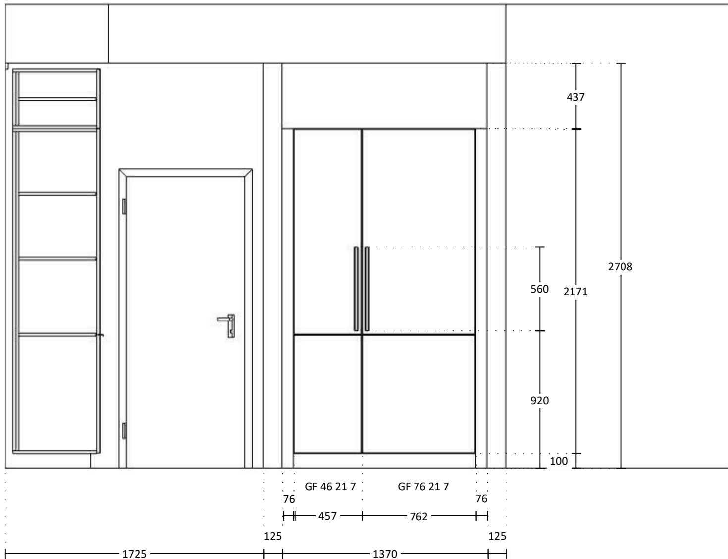
ELEVATION B
