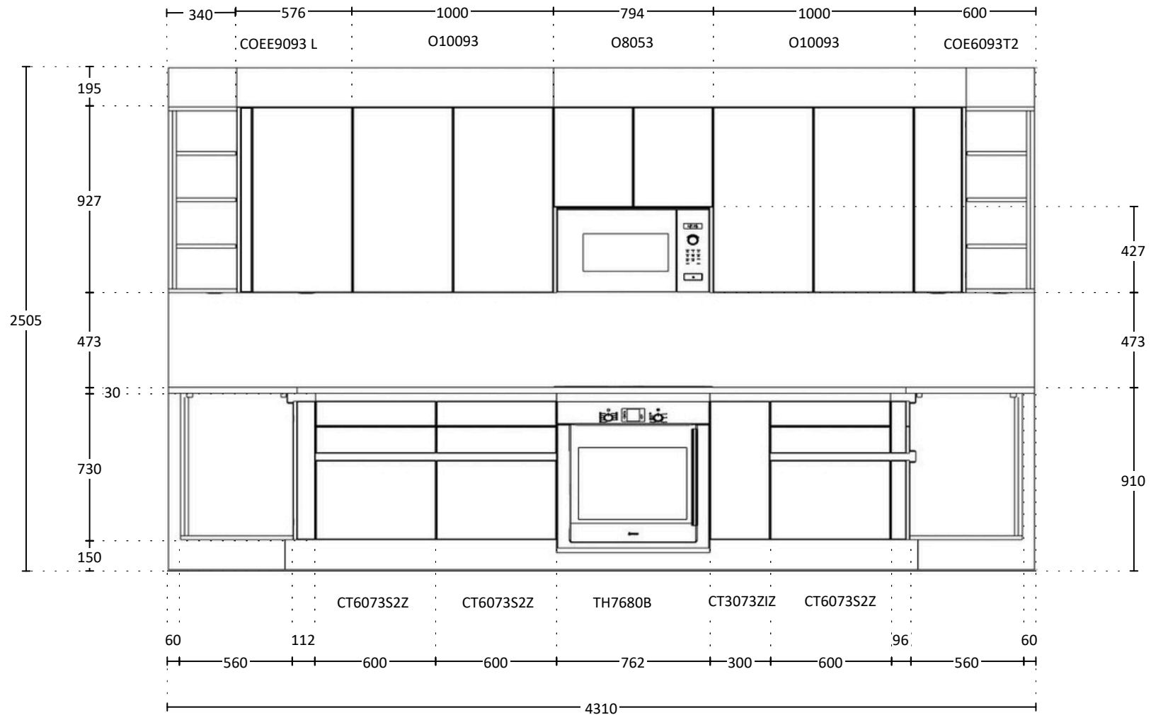
ELEVATION B
