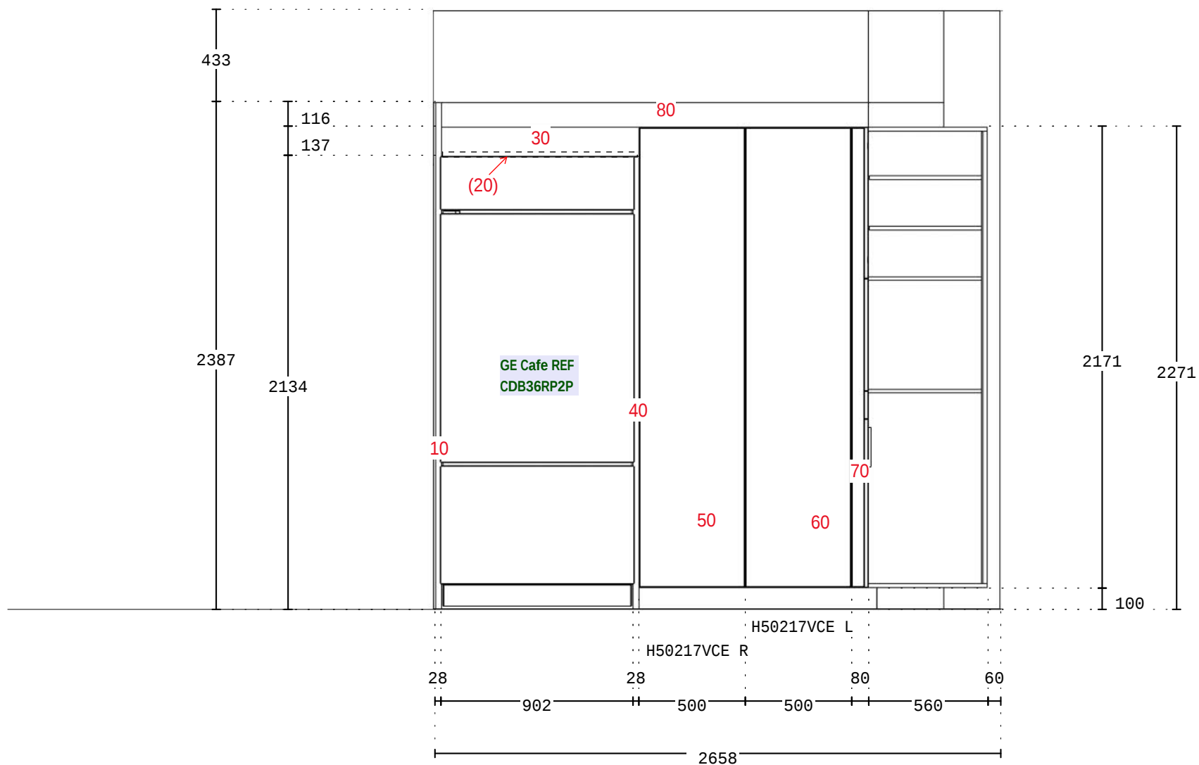
ELEVATION A
