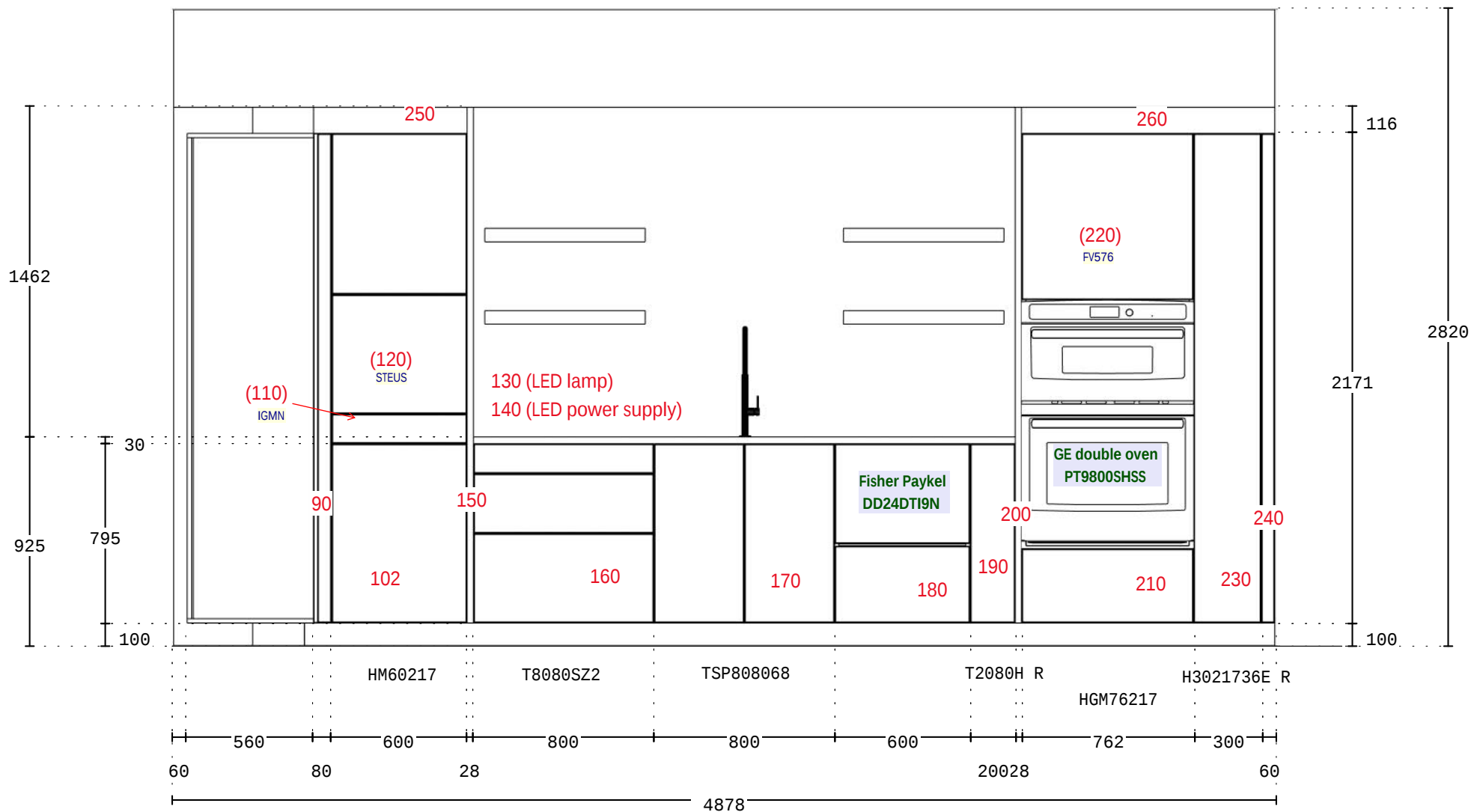
ELEVATION B
