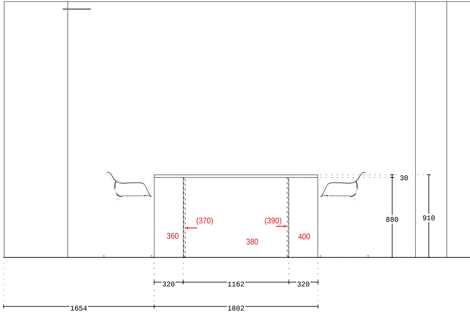
ELEVATION E
